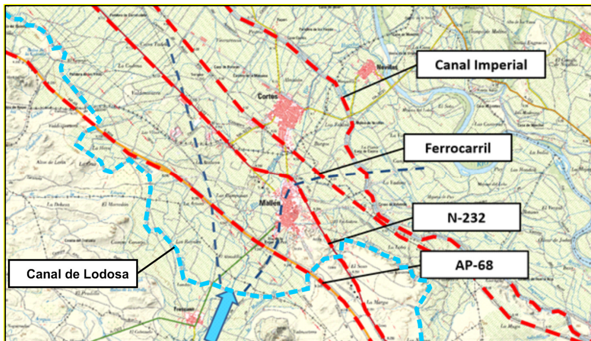
Figura 5. Infraestructuras transversales al río Huecha en el tramo de estudio (elaboración propia).
