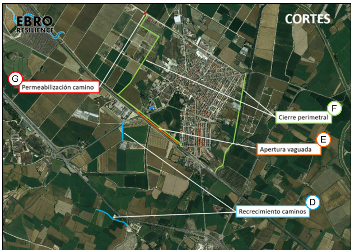
Figura 12. Alternativa propuesta en el entorno de Cortes (elaboración propia).
