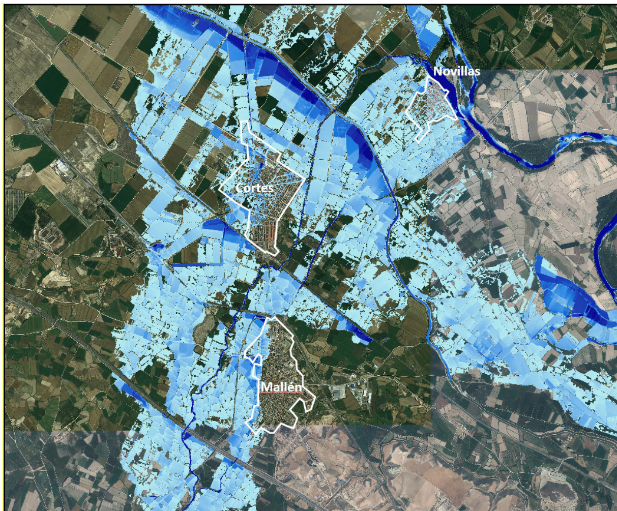
Figura 9. Resultados del modelo hidráulico para la avenida equivalente a la de septiembre de 2004 (elaboración propia).
